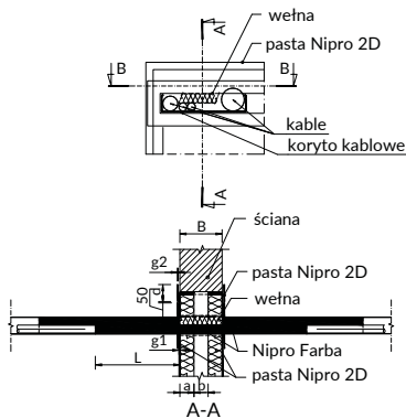
Rys. Zabezpieczenie przejść kabla lub wiązki kabli przez ścianę wykonane przy użyciu Nipro Farby i Pasty 2D.
