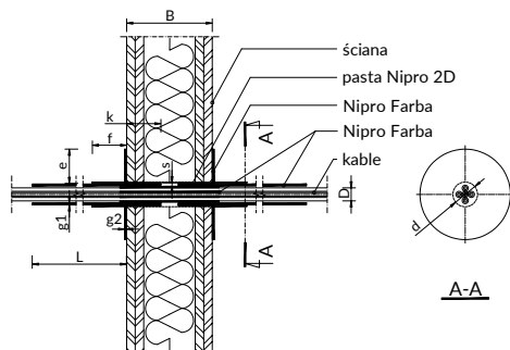
Rys. Zabezpieczenie przejść pojedynczego kabla lub wiązki kabli przez ścianę wykonane przy użyciu Nipro Farby i Pasty 2D.
