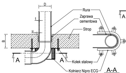
Rys. Przejście rury palnej przez strop z kolierzem Nipro ECG w kształcie U umieszczonym na kolanie rury.
