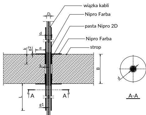
Rys. Zabezpieczenie przejść pojedynczego kabla lub wiązki kabli przez strop wykonane przy użyciu Nipro Farby i Pasty 2D.
