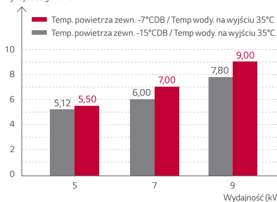
Wydajność grzewcza
