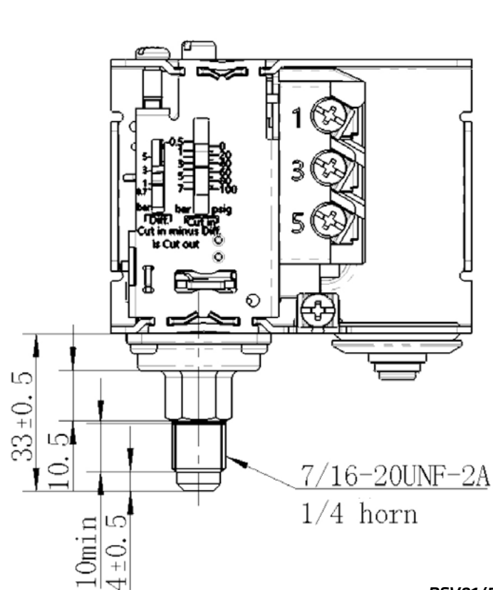
PSV01/50/60 \times L
