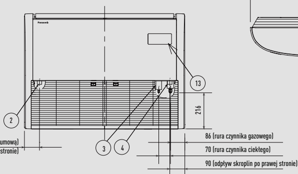
Polożenie otworów z tyłu jednostki wewnętrznej (na rysunku widok z przodu)
