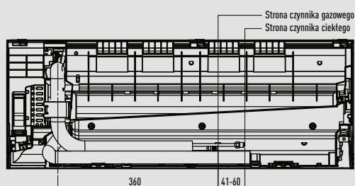
Polożenie jednostki wewnętrznej w stosunku do płyty montażowej
