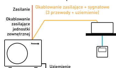
Jednostki PACi NX: metoda 3-przewodowa
