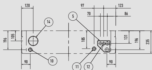
Polożenie otworu na rurę na powierzchni ściany (na rysunku widok z przodu)
