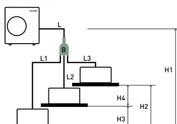
Split potrójny
