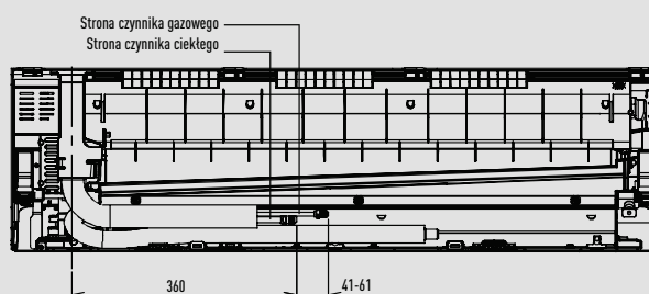
Polożenie jednostki wewnętrznej w stosunku do płyty montażowej
