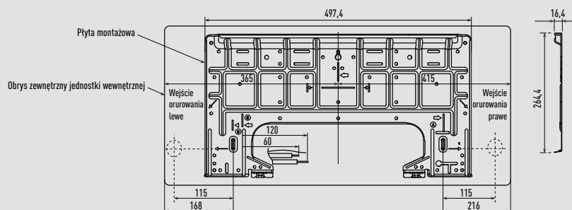
Polożenie jednostki wewnętrznej w stosunku do płyty montażowej
