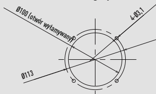
Widok szczegółowy przyłącza kanatu wlotowego powietrza
