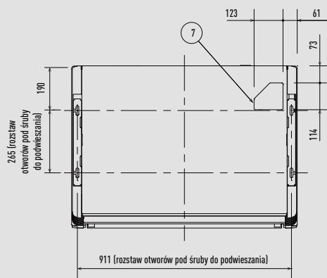
Widok szczegółowy przyłącza kanatu wlotowego powietrza
