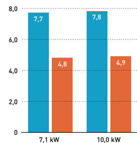
Sprawność sezonowa urządzeń serii PZH4
