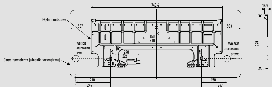
Położenie jednostki wewnętrznej w stosunku do płyty montażowej
