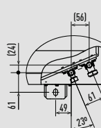
Widok A
