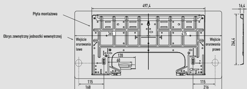
Położenie jednostki wewnętrznej w stosunku do płyty montażowej
