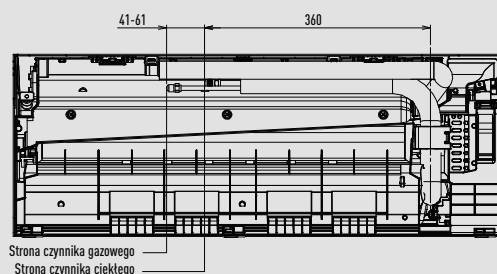
Położenie jednostki wewnętrznej w stosunku do płyty montażowej
