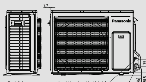
Zawór 3-drogowy po stronie czynnika gazowego (niskie ciśnienie)
