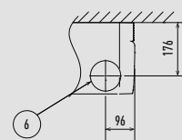
Polożenie otworu na rurę na powierzchni ściany (na rysunku widok z przodu)
