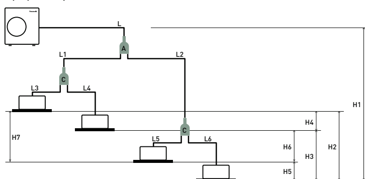
Split poczwórny
