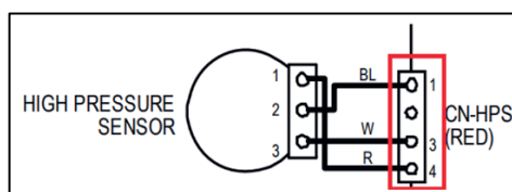
Złącze przetwornika HP CN-HPS
