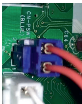
Złącze presostatu HP CN-PSW1
