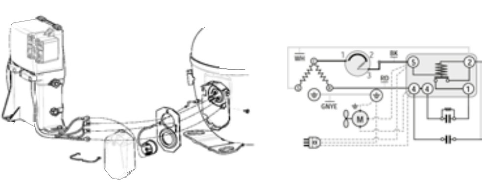
SM21 - UNT SERIE CSR BOX
