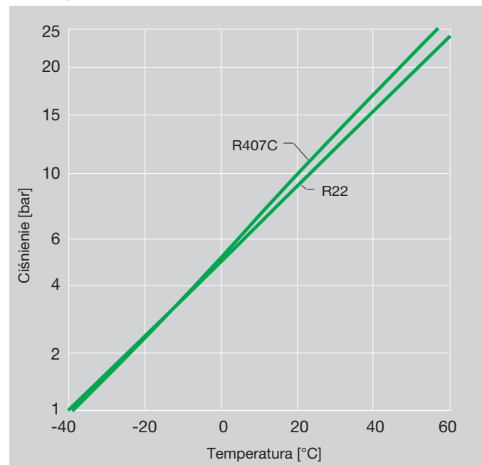
Rys. 22. Porównanie parametrów nasycenia czynników R407C i R22
