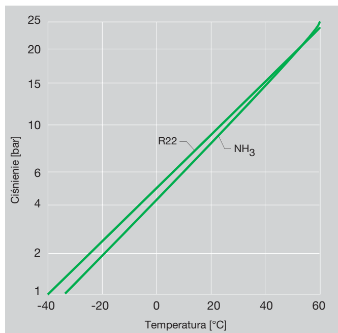
Rys. 26/2. Porównanie parametrów nasycenia amoniaku i czynnika R22
