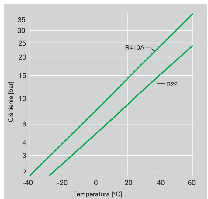
Rys. 23/2 Porównanie parametrów nasyceń czynników R410A i R22
