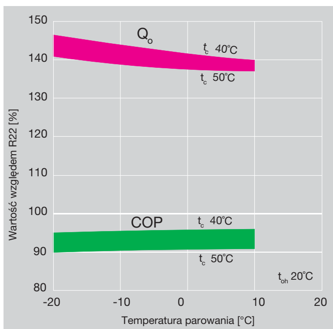
Rys. 23/1 Porównanie wydajności chłodniczej ( Q_o ) i współczynnika wydajności chłodniczej (COP) czynników R410A i R22 w instalacji ze sprężarką półtermetyczną, w zależności od temperatury parowania i temperatury skraplania ( t_c )
