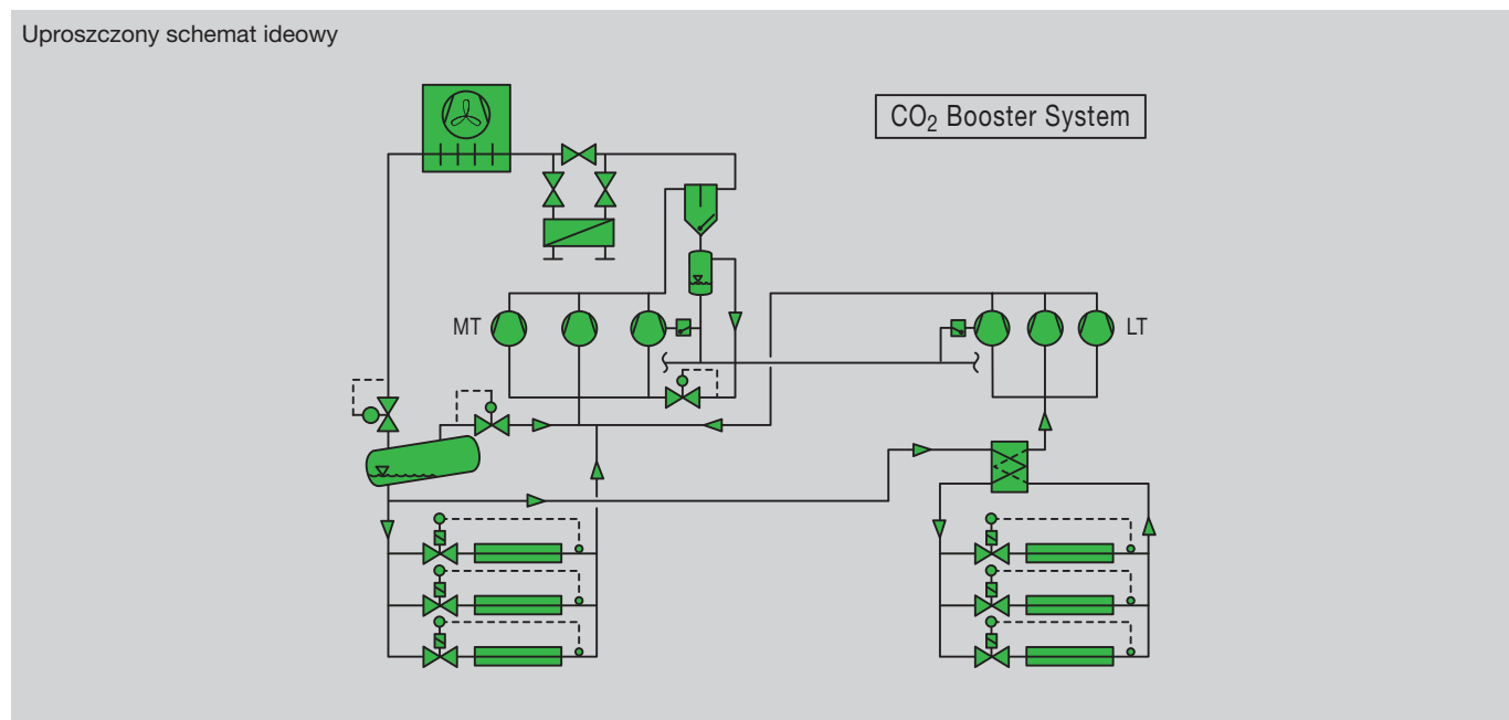
Rys. 31. Schemat ideowy przykładowego nadkrytycznego układu chłodniczego z CO 2
