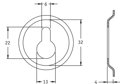
Asole di fissaggio Fixing slots
